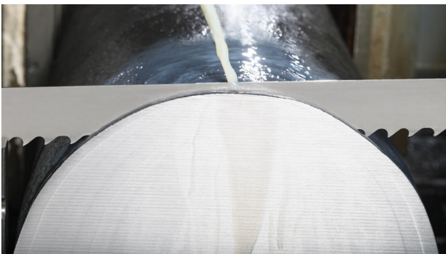
Figura 1: Uso flexible: La nueva sierra de cinta con inserciones de metal duro MARADUR ® de WIKUS también es indicada para máquinas sin paquete de metal duro. Fuente: WIKUS-Sägenfabrik
